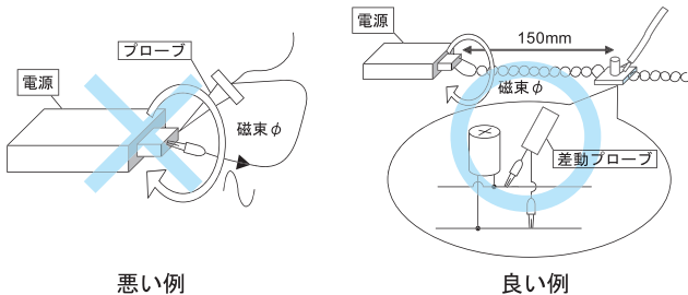
悪い例 良い例 図1.2 出力リップル・リップルノイズ測定例
