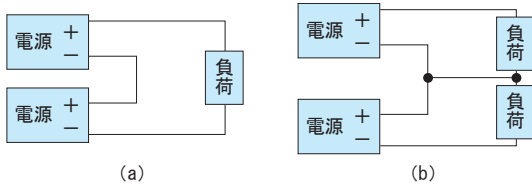
図2.1 直列運転時の接続例
