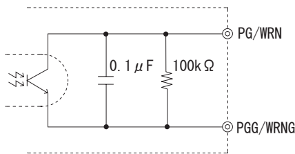
図 1.5 PG/WRN 信号内部回路
